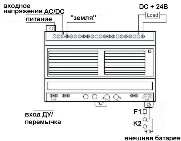
Схема подключения источника бесперебойного питания
