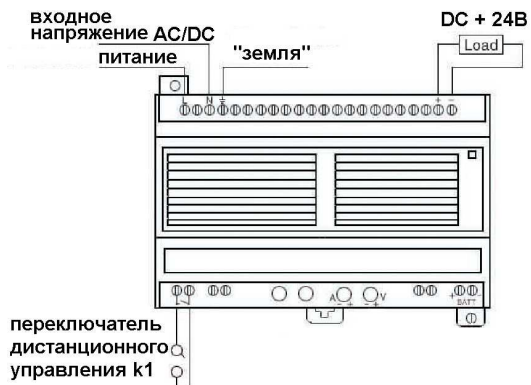
Схема подключения дистанционного управления
