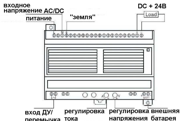
Схема подключения
