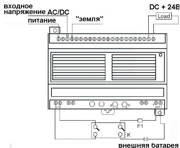
Схема подключения источника бесперебойного питания и дистанционного управления
