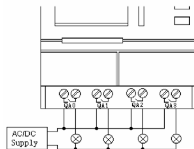
Рис.2.11 Подключение релейных выходов.
