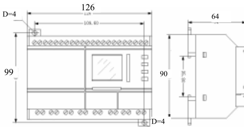
Рис.2.3 Установочные размеры контроллера SR-22xxxx
