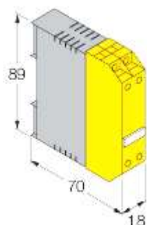
Габаритные размеры
