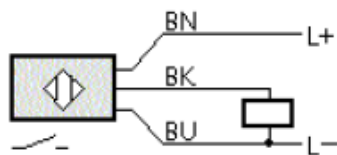
Схема подключения
