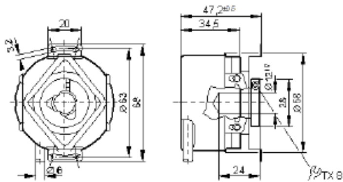
Габаритный чертёж
